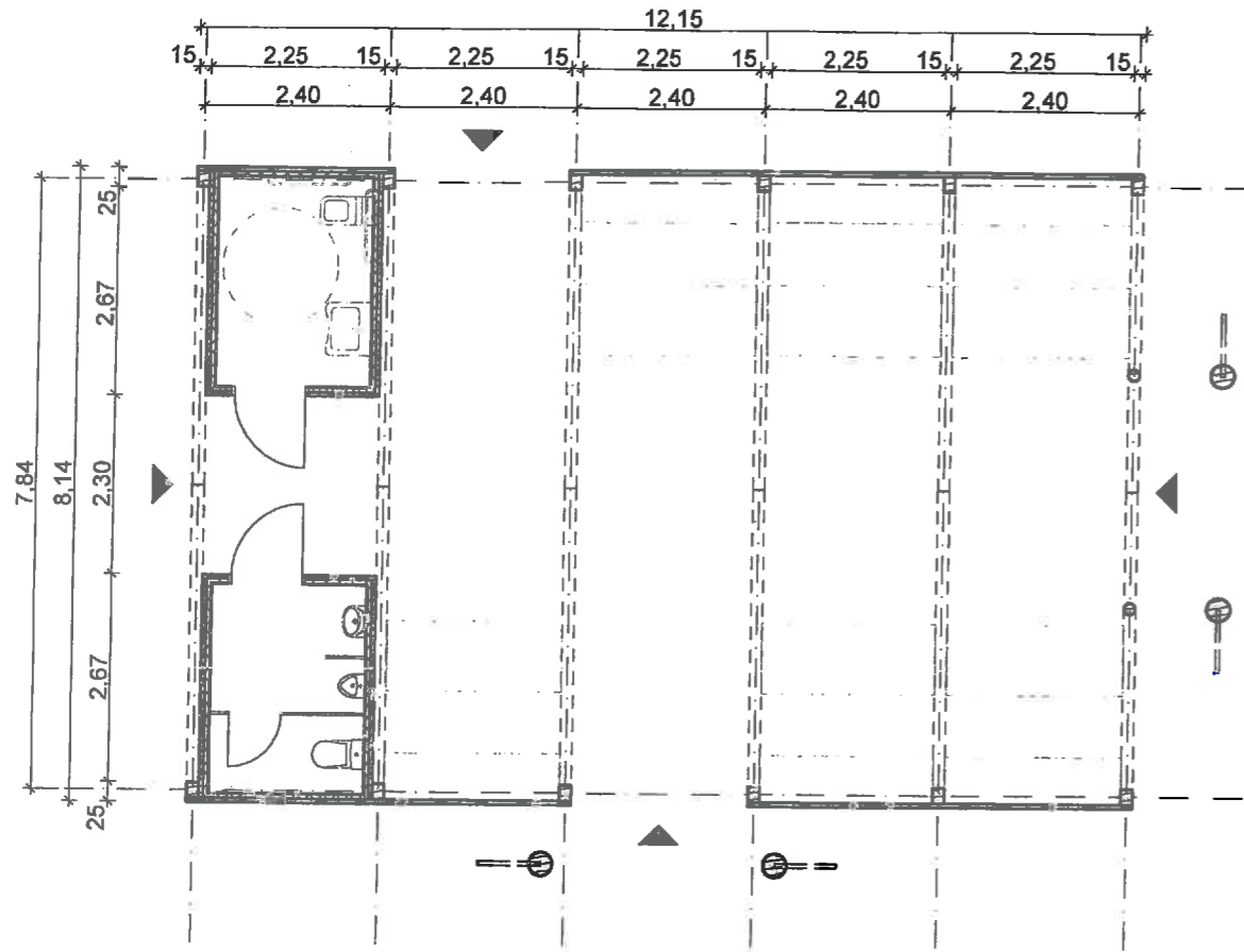
Alaprajz _ 1:100
